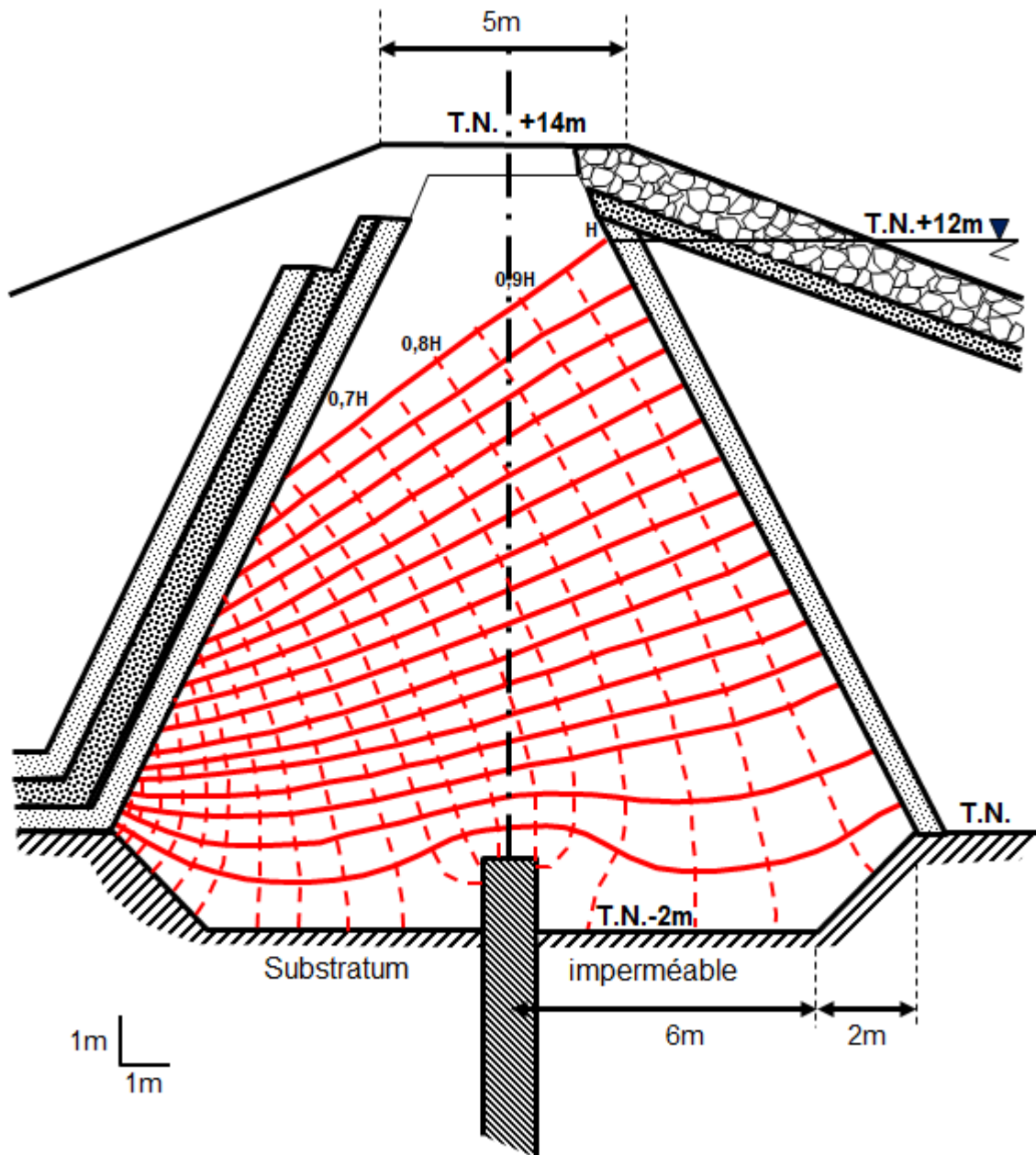
Figure 2. Réseau d'écoulement à travers le noyau du barrage
